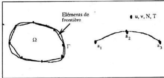
Figure 2 : Discretisation de la frontière en éléments quadratiques.
