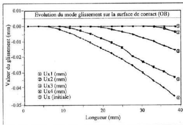
Figure 8 : Evolution de la distribution des déplacements tangentiels sur la surface de contact (OB), pour \lambda = 1 , F_2 = 5 \text{ daN/mm} et F_1 = (5, 10, 15, 20 \text{ daN/mm}) .
