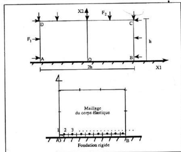
Figure 5 : Cas de chargement et maillage.
