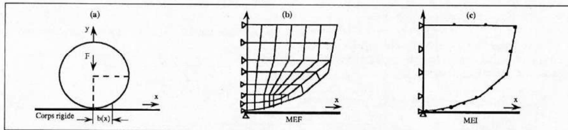
Figure 3 : Analyse du problème de Hertz.
