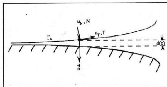
Figure 1 : Contact entre un corps élastique et une fondation rigide.
