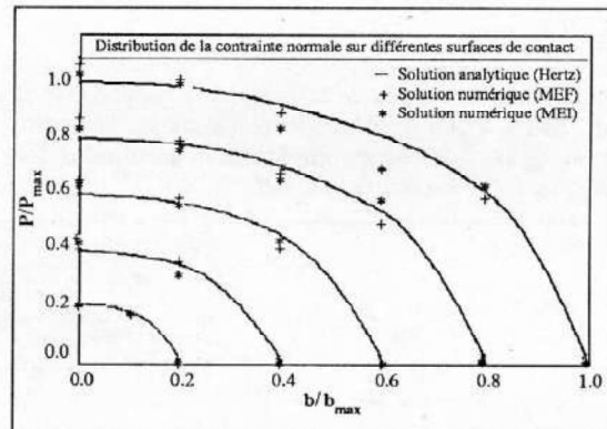
Figure 4 : Courbes comparatives. Distribution de la contrainte normale sur la surface de contact.
